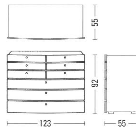
Kommode 7, 3 breite und 6 schmale Schubladen.
